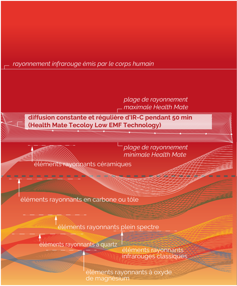
Émissions spectrales à puissance de rayonnement maximale
